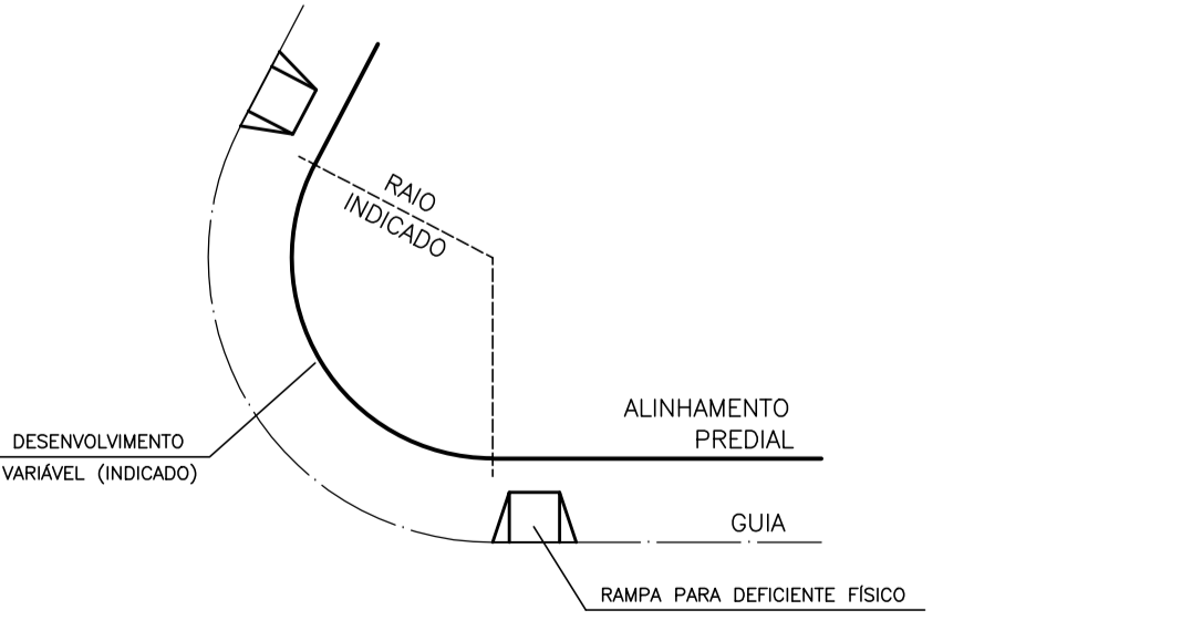
DETALHE DE CONCORDÂNCIA DE ALINH. PREDIAL IRREGULAR ESCALA 1:250
